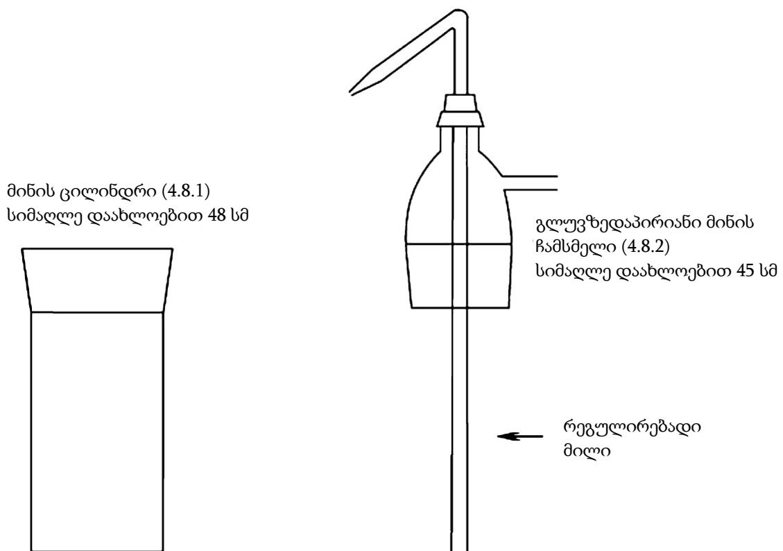
სურათი 1: ექსტრაქციის აპარატი (ამ თავის პუნქტი 4.8)
