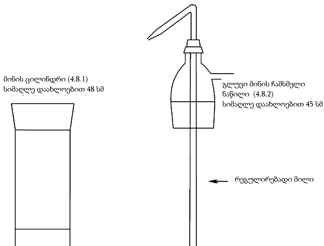
სურათი N1: ექსტრაჰირების აპარატი (ამ თავის პუნქტი 4.8)
